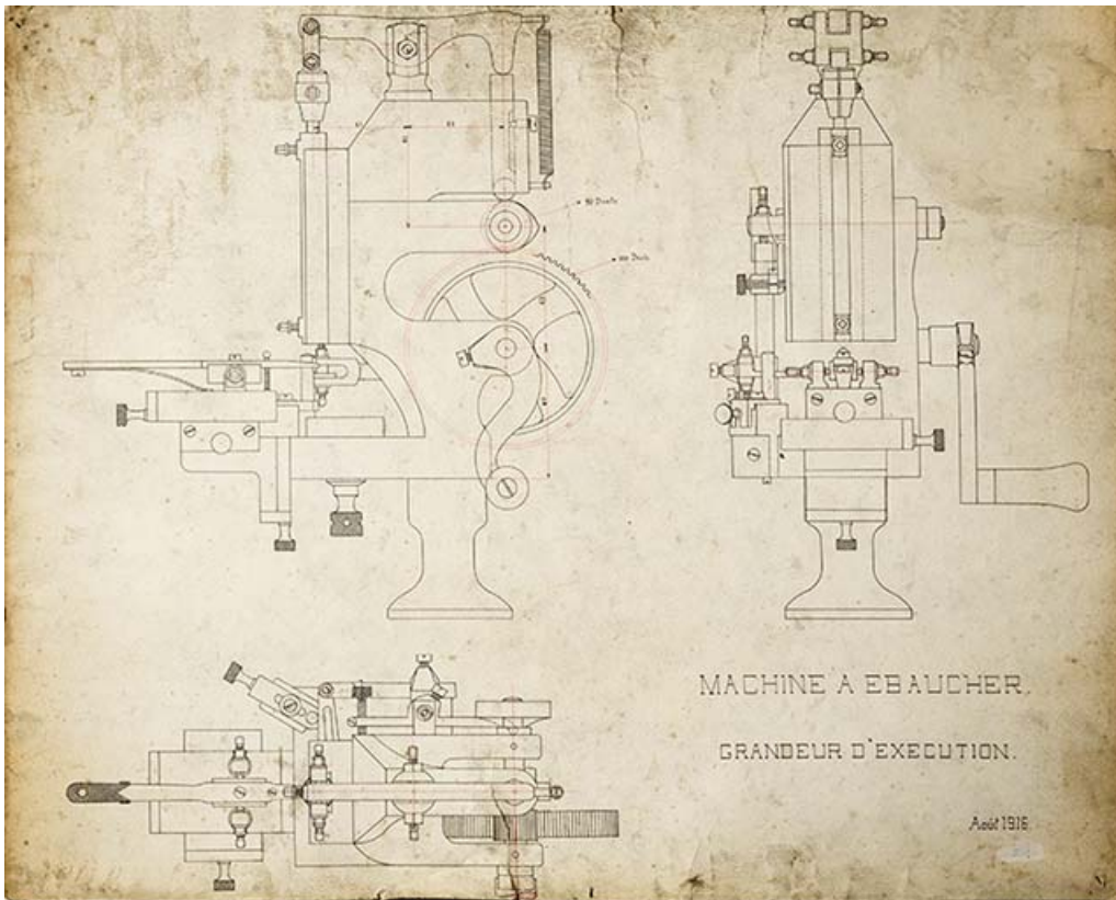
Machine à ébaucher. Grandeur d'exécution, août 1916. 25, Maïche, 13 rue Sous Montjoie
