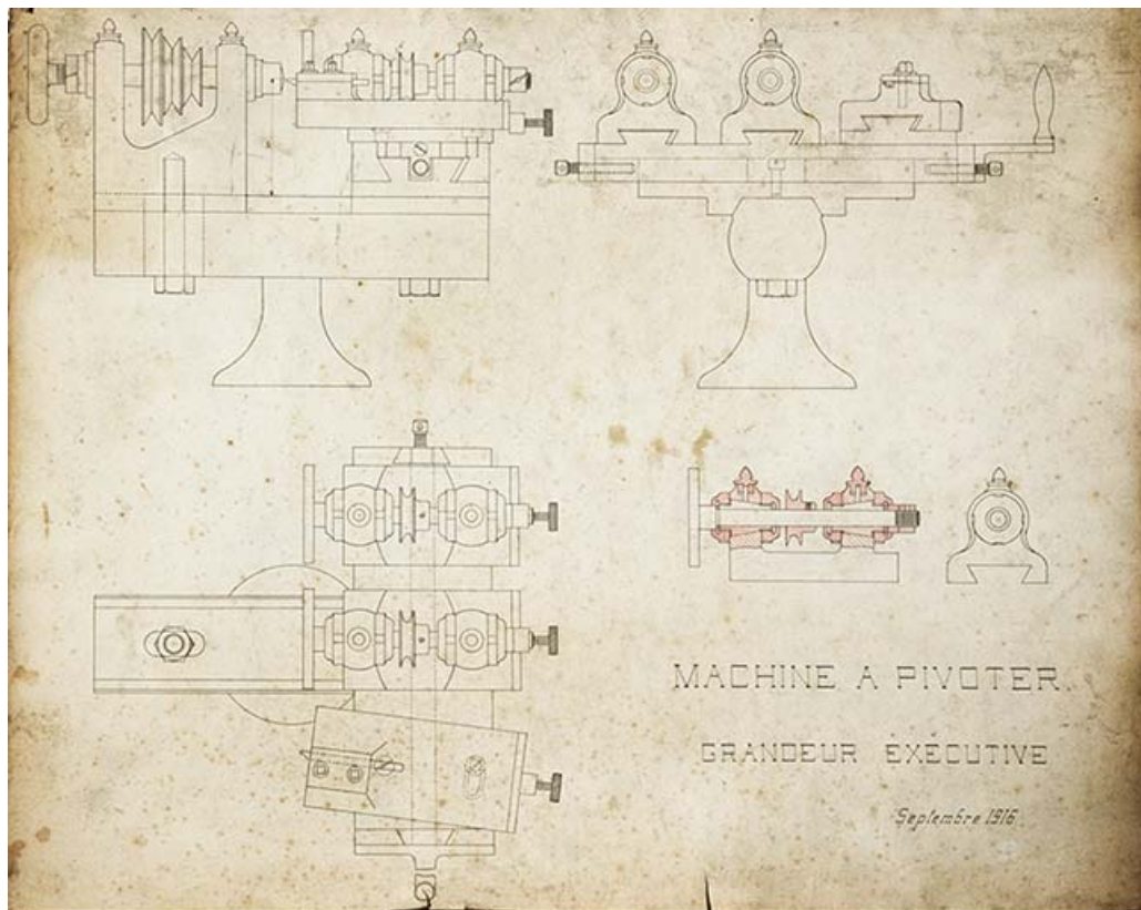
Machine à pivoter. Grandeur exécutive, septembre 1916. 25, Maïche, 13 rue Sous Montjoie
