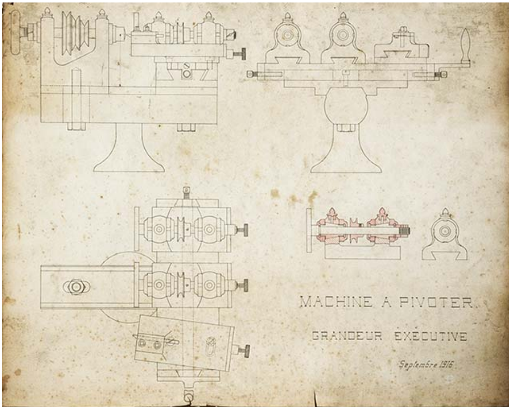
Machine à pivoter. Grandeur exécutive, septembre 1916. 25, Maîche, 13 rue Sous Montjoie
