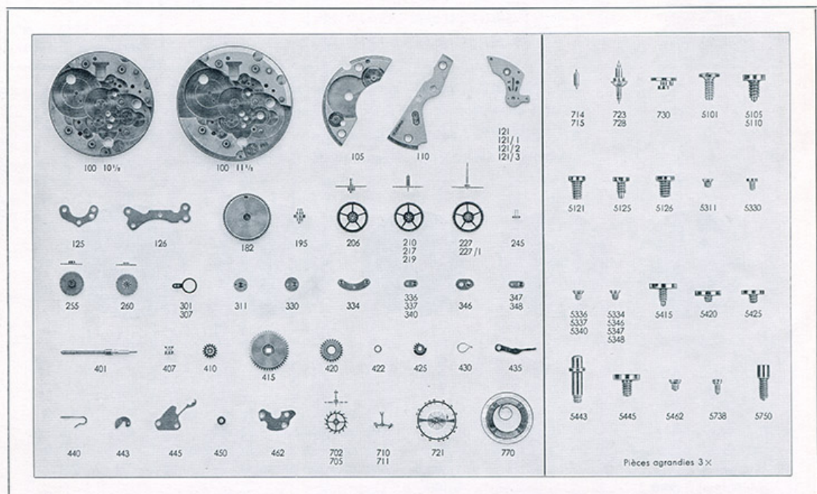
Calibres [jeambrun] 10 1/2''' - 23 D [et] 11 1/2''' - 26 D - 15 à 21 rubis [éclaté des fournitures], 1973. 25, Charquemont, 12 Rue Neuve
