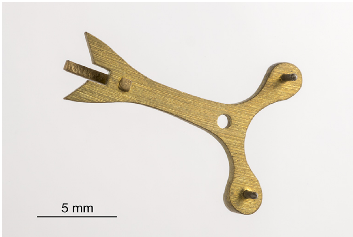
Echappement à chevilles : ancre (les chevilles sont visibles à droite). 25, Charquemont, 12 Rue Neuve
