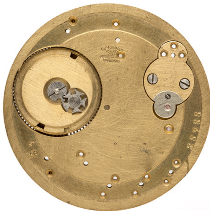
Platine nue, vue du côté cadran. Noter le barillet et son système d'arrêtage (croix de Malte) à gauche, le chariot à droite. 25, Charquemont, 12 Rue Neuve
