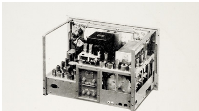
Le chassis du 2 e changeur de fréquence, est représenté non muni de son capot de blindage.
