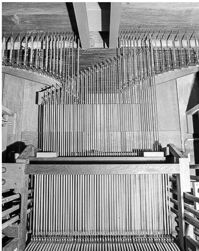
Mécanique vue de face.
