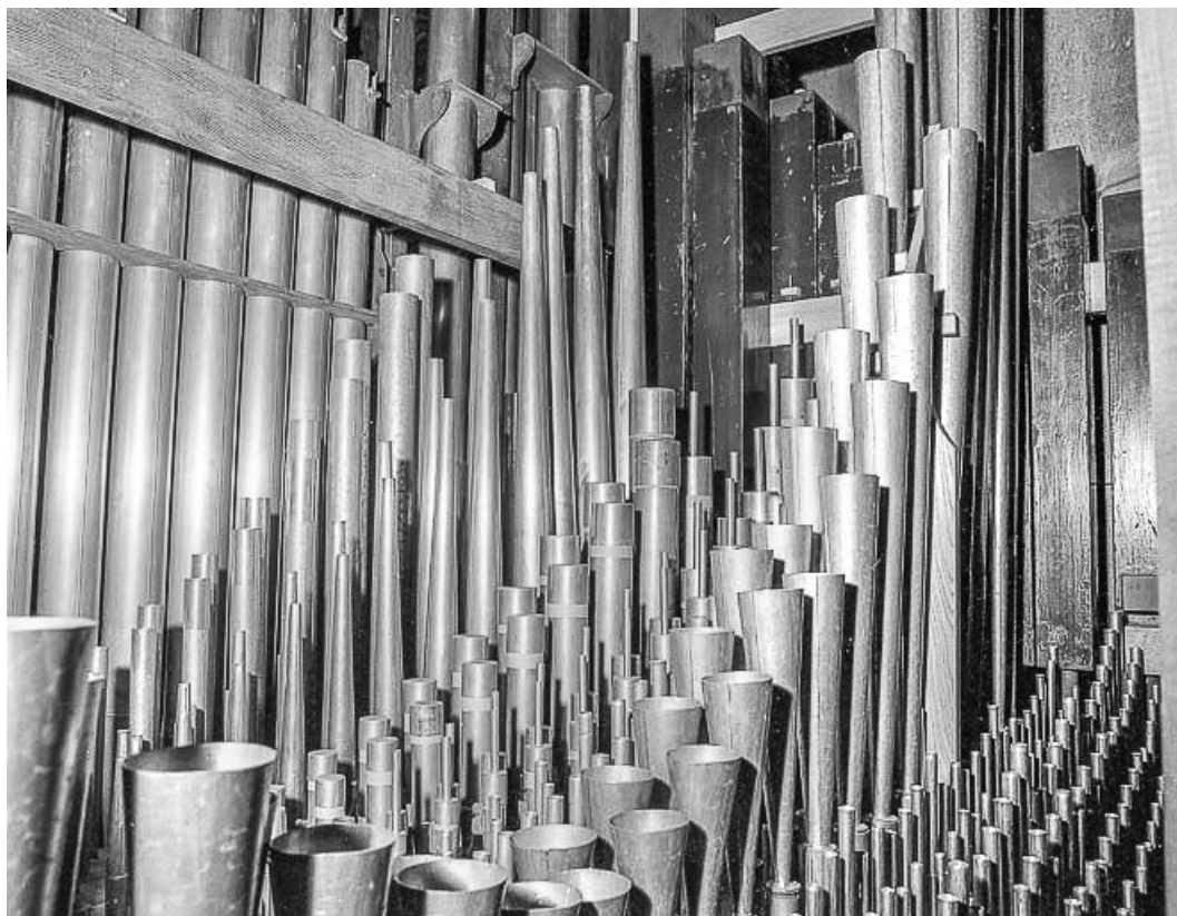
Tuyauterie vue de trois quarts gauche.
