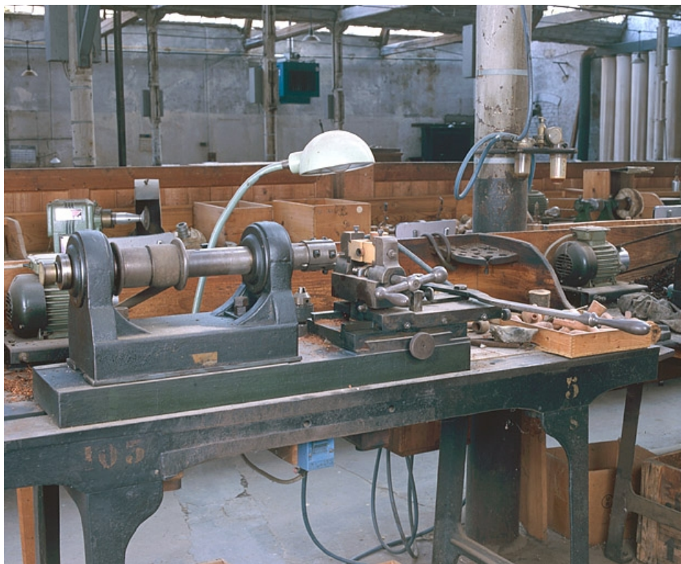
Vue d'ensemble rapprochée de la machine de gauche (atelier principal). 25, Baume-les-Dames rue des Pipes, lieudit : Gondé
