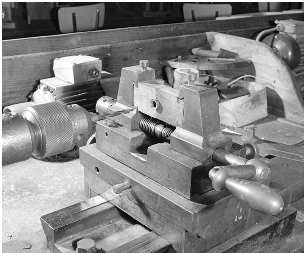
Le chariot mobile et le mandrin porte-mèche, de trois quarts gauche (atelier principal). 25, Baume-les-Dames rue des Pipes, lieudit : Gondé
