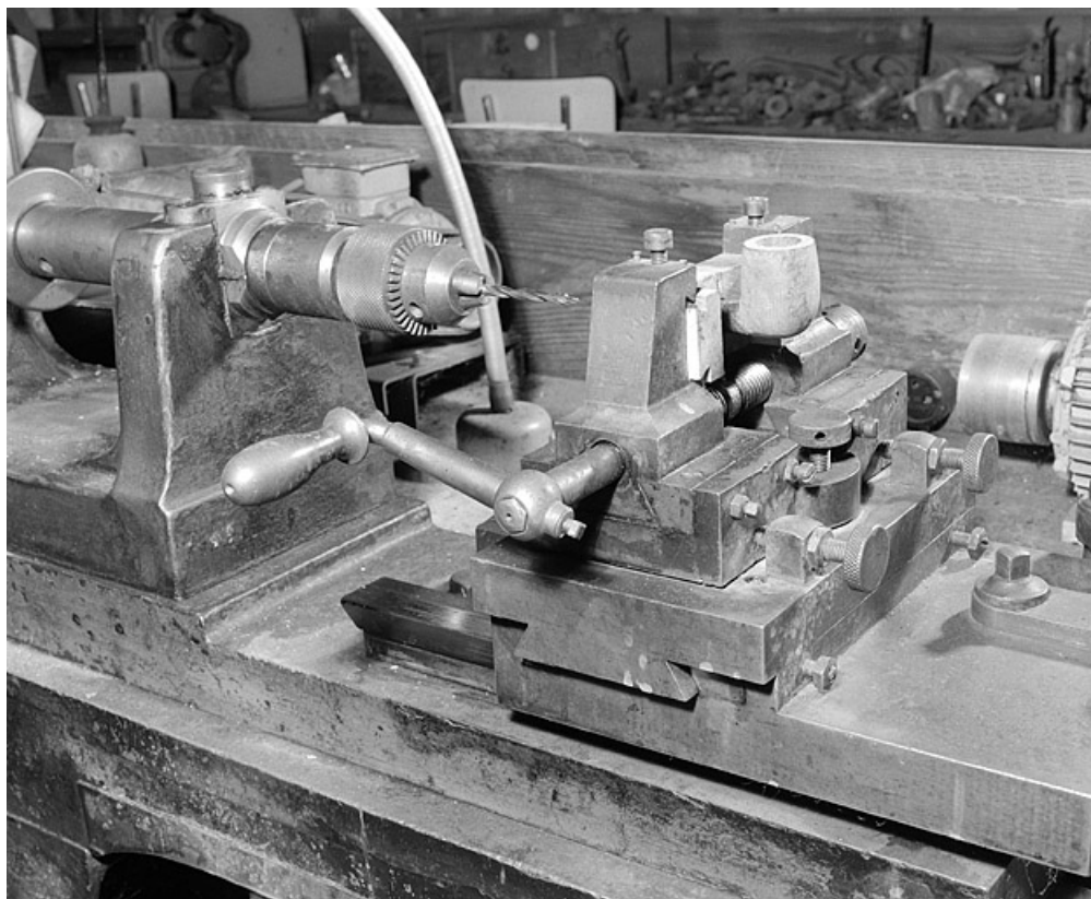
Le chariot mobile et le mandrin porte-mèche, de trois quarts droite (atelier principal). 25, Baume-les-Dames rue des Pipes, lieudit : Gondé
