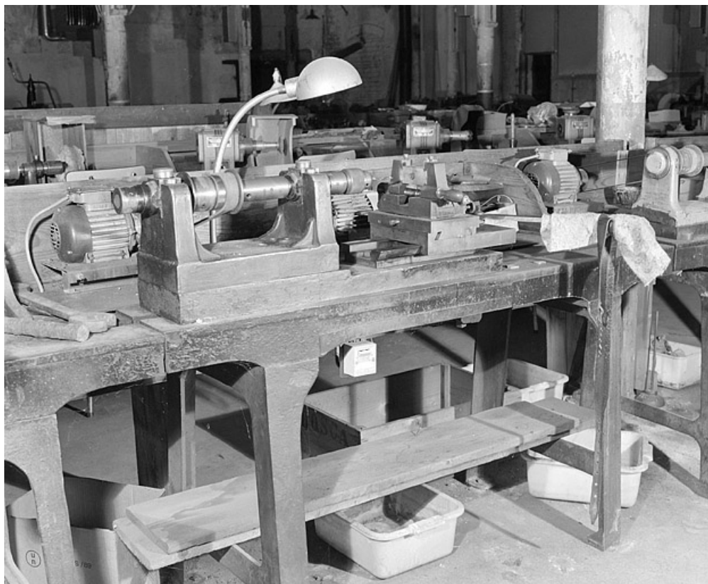
Vue d'ensemble d'une des machines encore munie de sa ceinture (atelier principal). 25, Baume-les-Dames rue des Pipes, lieudit : Gondé
