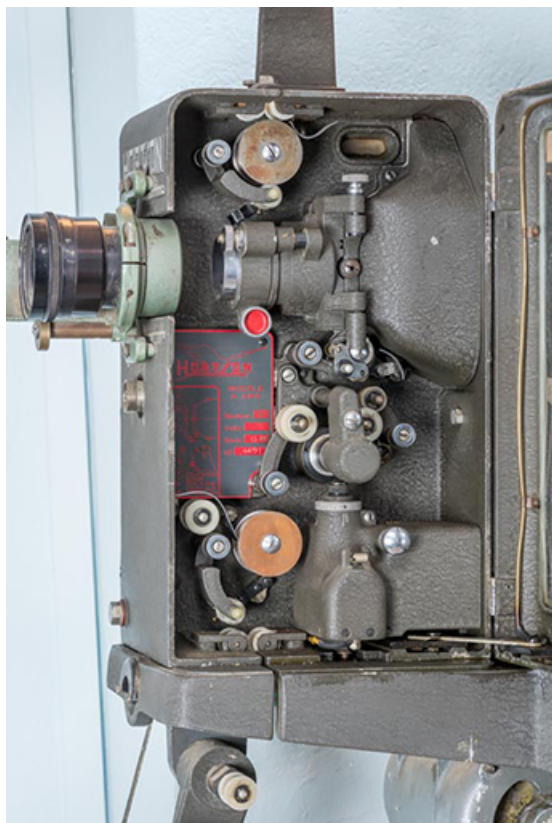
Mécanisme projecteur (système d'entraînement du film et objectif). 21, Lacanche rue de l' Église
