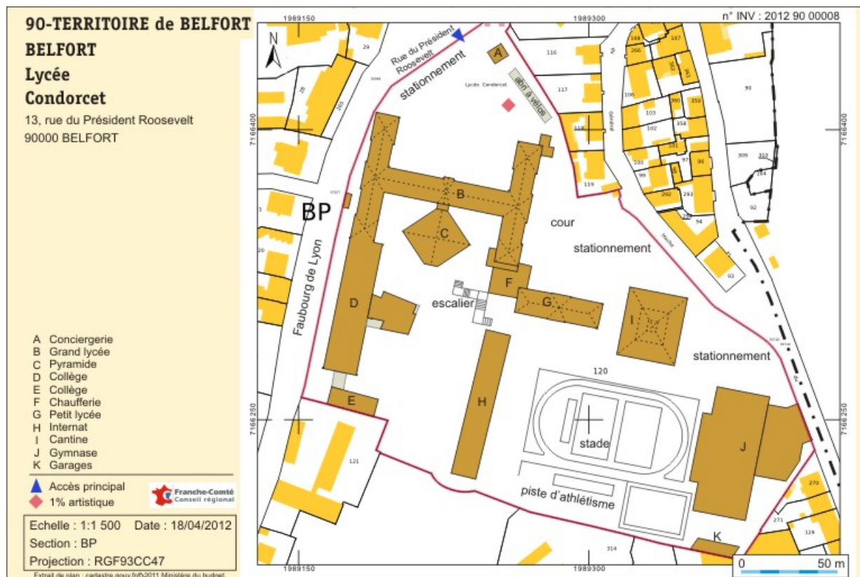
Plan-masse et de situation. Extrait du plan cadastral numérisé, section BP, échelle 1:1500. 90, Belfort, 13 rue du président Roosevelt
