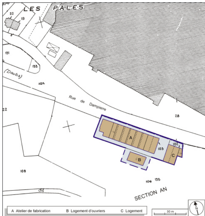
Plan-masse et de situation. Extrait du plan cadastral, 1984, section AN, 1:1000. 90, Beaucourt, 1 rue de Dampierre
