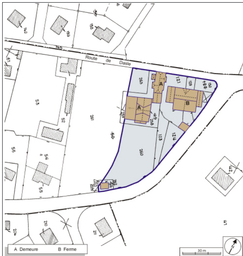
Plan-masse et de situation. Extrait du plan cadastral, 1984, section AM, 1:1000.
