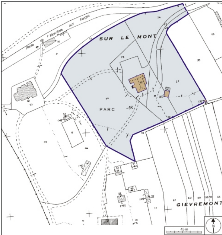
Plan-masse et de situation. Extrait du plan cadastral, 1984, section B, 1:1000 réduit à 1:1500. 90, Morvillars, 9 rue des Forges
