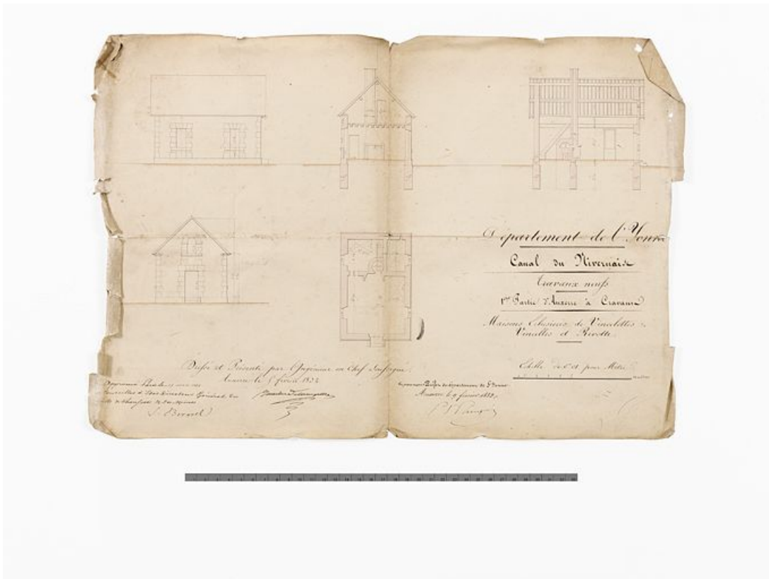
"Maisons éclésières de Vincelottes, Vincelles et Rivotte". Élévation, plan et coupe. (VNF-direction territoriale Centre-Bourgogne ; subdivision de Corbigny)
