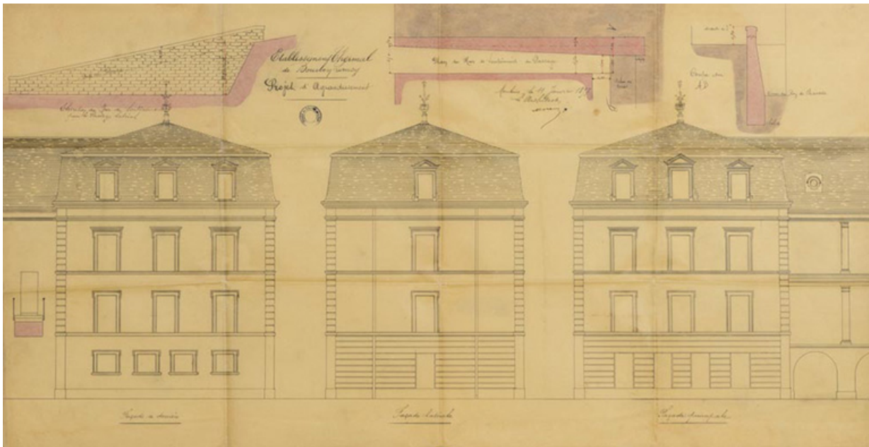
Projet de pavillon annexe, par l'architecte René Moreau (11 janvier 1897), façades. 71, Bourbon-Lancy, 2 Parc thermal
