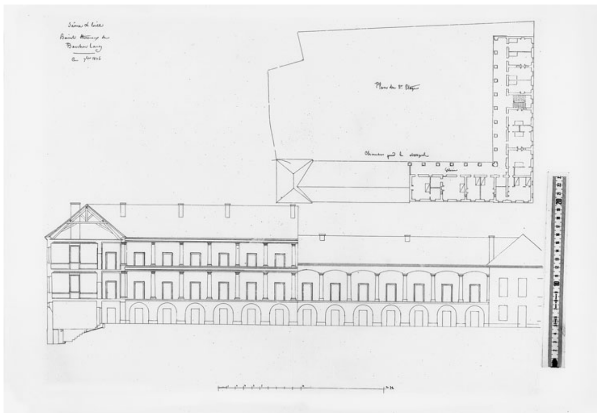
Projet de François Agnéty présenté au Conseil des Bâtiments civils en septembre 1836, élévation et plan du second étage. 71, Bourbon-Lancy, 2 Parc thermal
