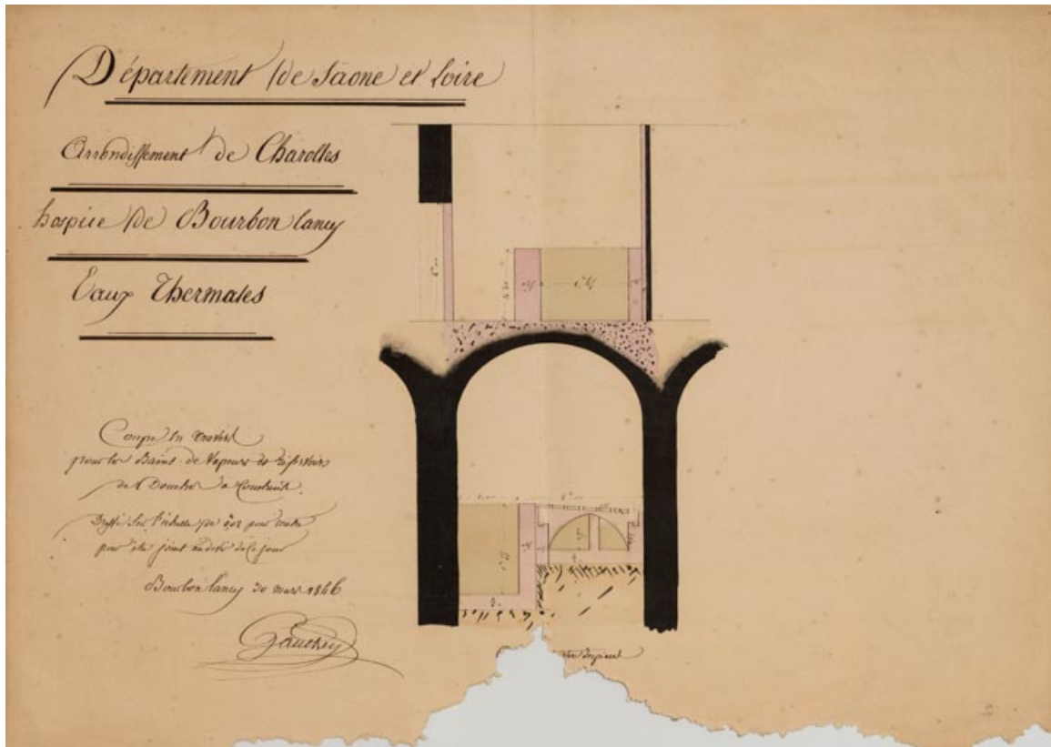
Projet pour la construction d'un bain de vapeur, coupe du rez-de-chaussée et de l'étage (1846). 71, Bourbon-Lancy, 2 Parc thermal
