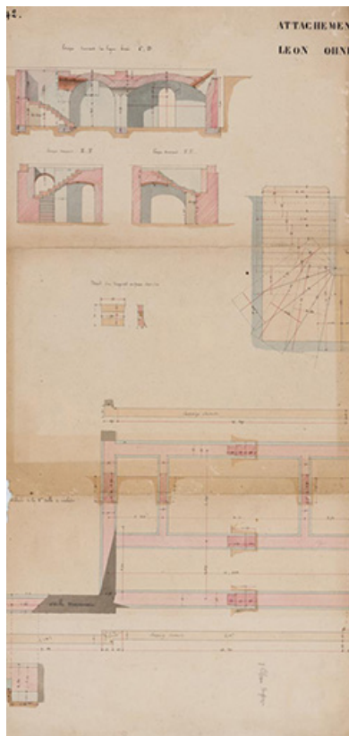
Dessin de Léon Ohnet en lien avec l'établissement thermal (?). 71, Bourbon-Lancy, 2 Parc thermal
