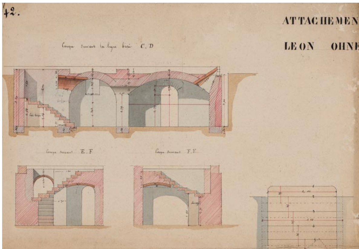
Dessin de Léon Ohnet en lien avec l'établissement thermal (?). 71, Bourbon-Lancy, 2 Parc thermal
