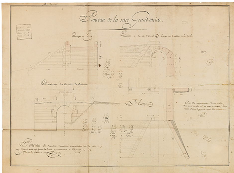
Plan, coupe, élévation. Ponceau de la raie Grand-meix. Dessin, sans date [1841 ?].
