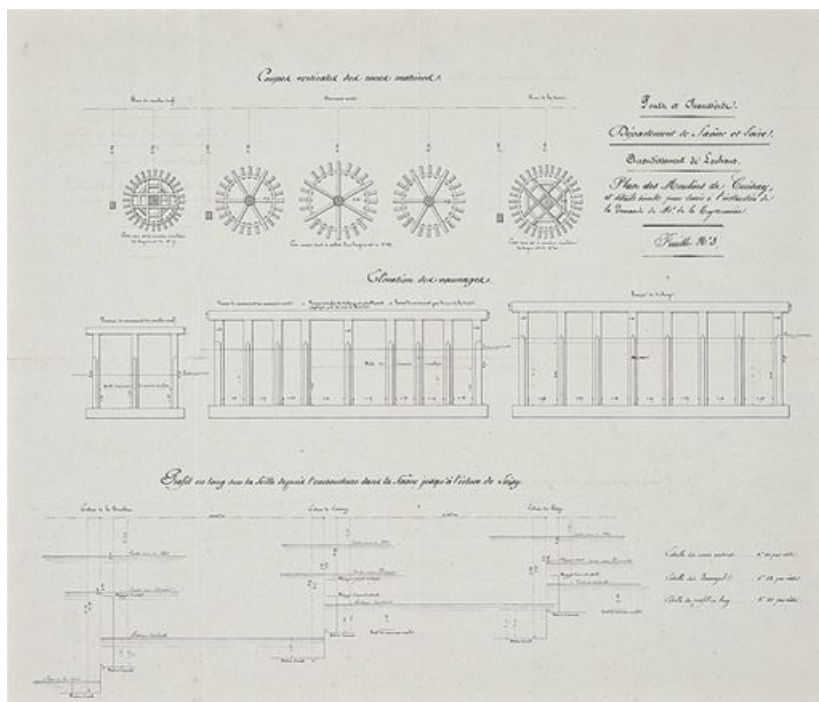
"Plan des moulins de Cuisery et détails divers pour servir à l'instruction de la demande de M. de la Teysonnière, feuille n° 3 coupes verticales des roues motrices, élévation des vannes, profil en long depuis l'embouchure dans la Saône jusqu'à l'écluse de Loisy". Sans doute vers 1842. (Dessin, Archives VNF-direction territoriale Centre-Bourgogne ; subdivision de Montceau-les-Mines) 71, Cuisery
