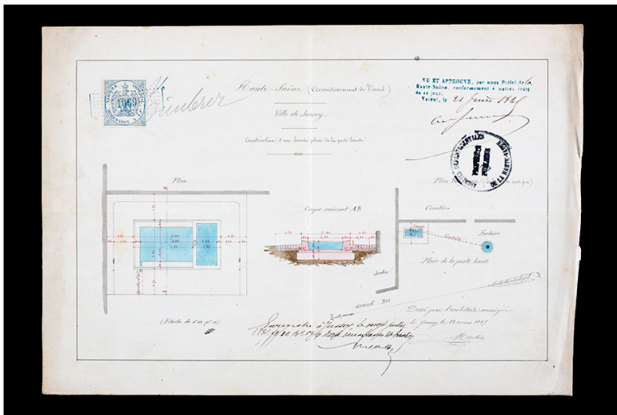
Plan et coupe projetés du lavoir de la porte haute de Jussey, 1865. 70, Jussey rue Charles-Bontemps
