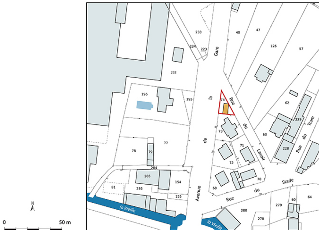
Plan-masse et de situation. Extrait du plan cadastral numérisé de la direction générale des finances publiques, 2025, 1/1 000. 70, Jussey avenue de la Gare, lieudit : la gare
