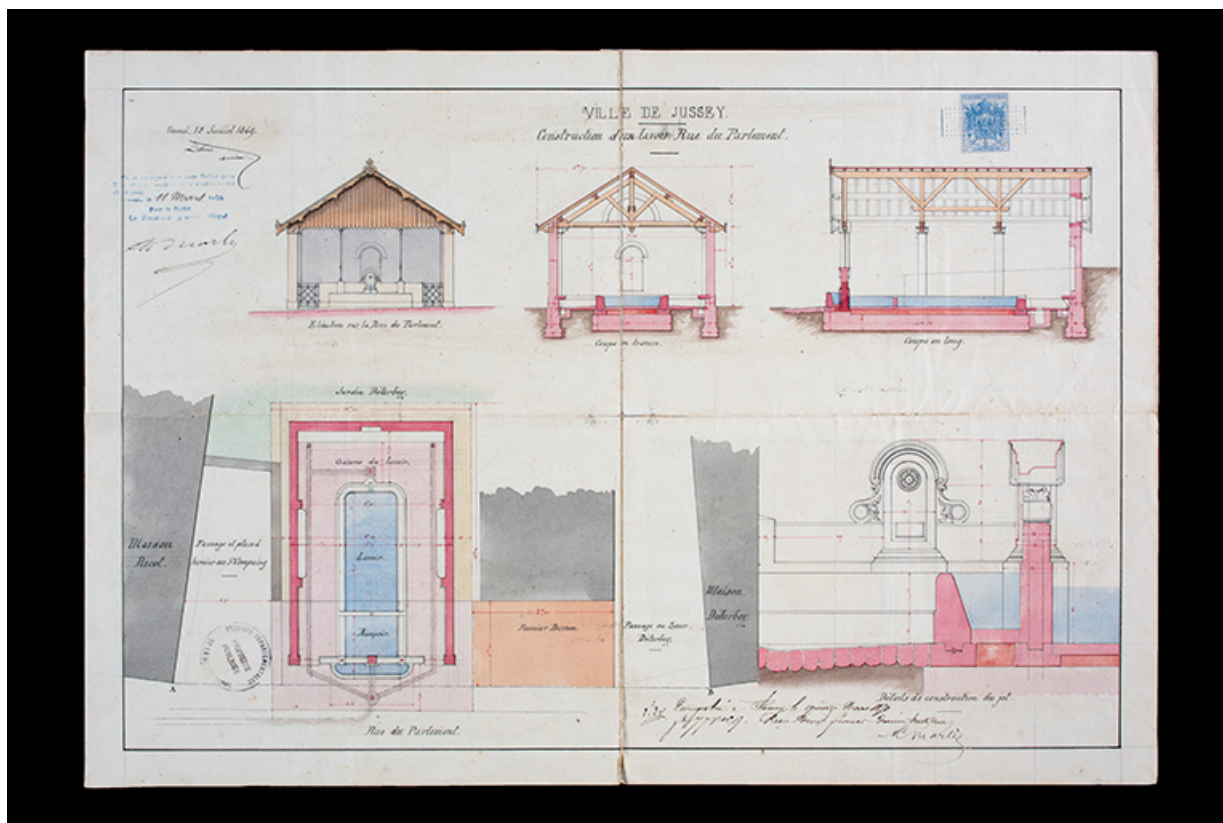
Plan, élévations, coupes et vue de détail de la fontaine-lavoir rue du Parlement à Jussey, 1869. 70, Jussey rue du Parlement
