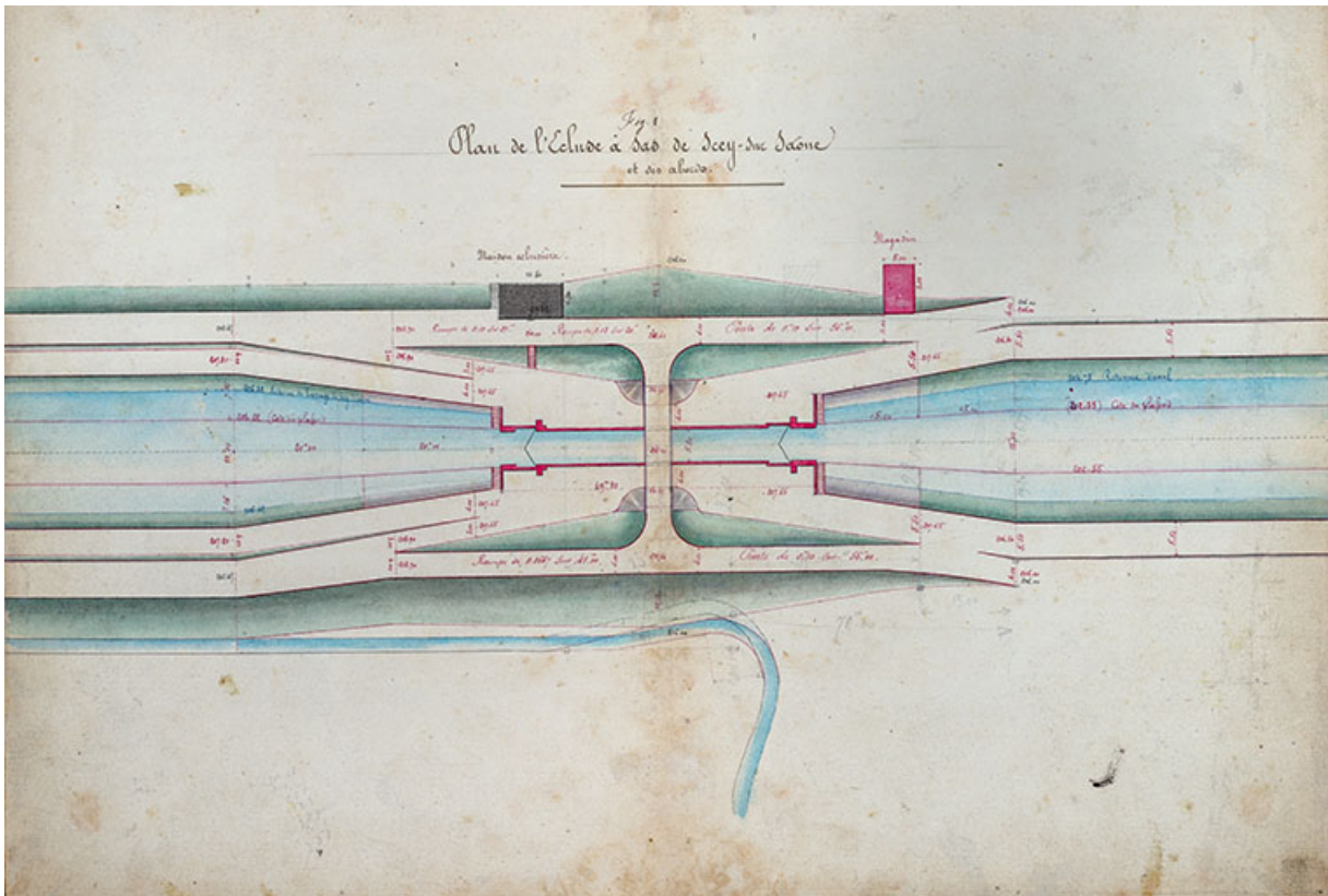
Achèvement de la dérivation de Scey-sur-Saône, écluse à sas - Plans, élévations, coupes et détails (1876). 70, Chassey-lès-Scey, 3 écluse de Chassey
