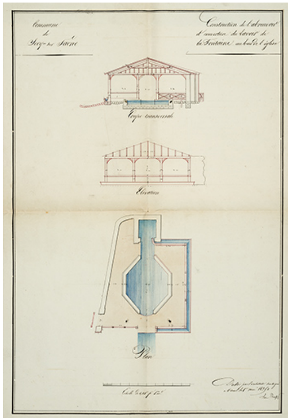
Le Beuffe. Construction de l'abreuvoir et couverture du lavoir de la fontaine au bas de l'église. 1835. 70, Scey-sur-Saône-et-Saint-Albin rue de la Fontaine Larie
