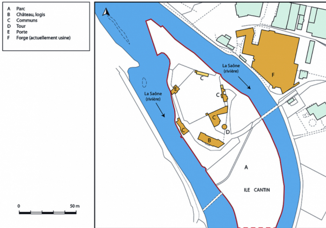
Plan-masse et de situation. Extrait du plan cadastral, 2019. 70, Conflandey
