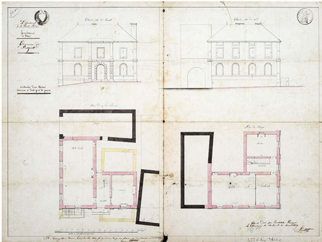
Plans et élévation du projet de construction de la mairie-école, 1839. 70, Purgerot, 2 rue des Bournaux
