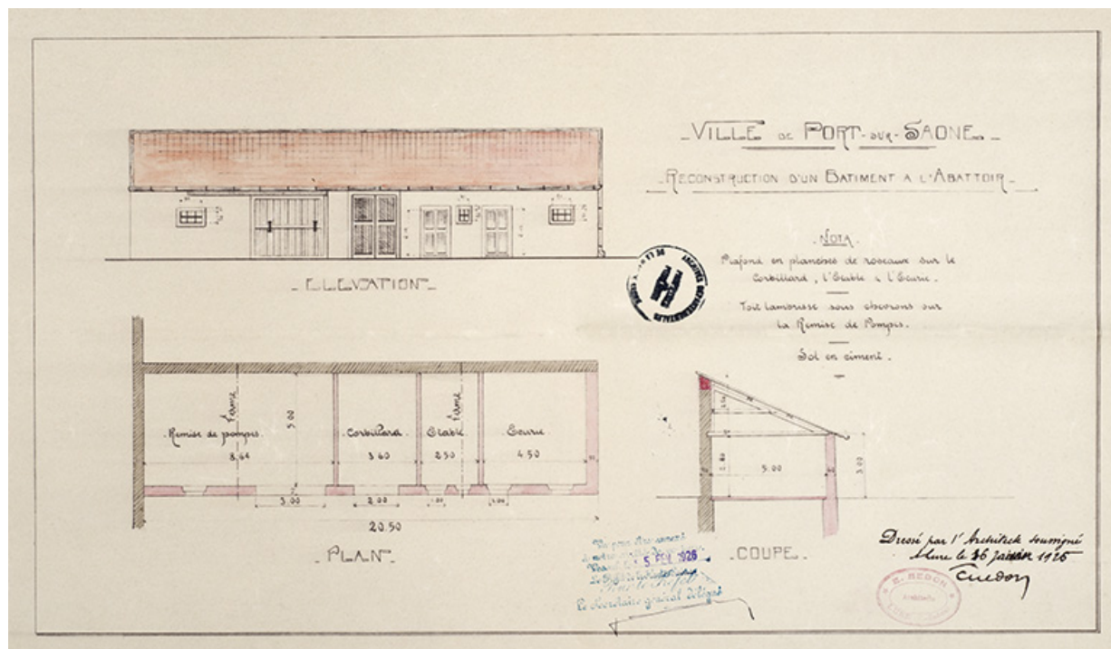
Reconstruction d'un bâtiment à l'abattoir : plan, coupe et élévation.
