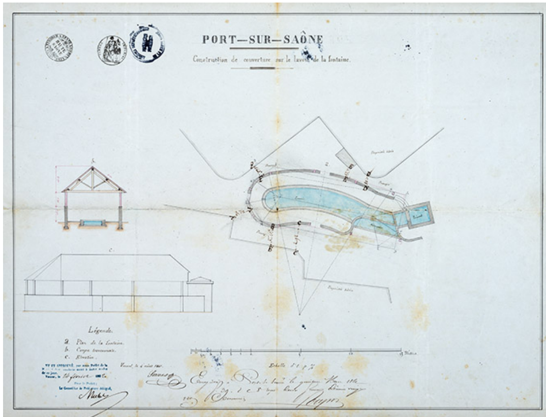
Plan pour la couverture à construire, 1861. 70, Port-sur-Saône rue de la fontaine
