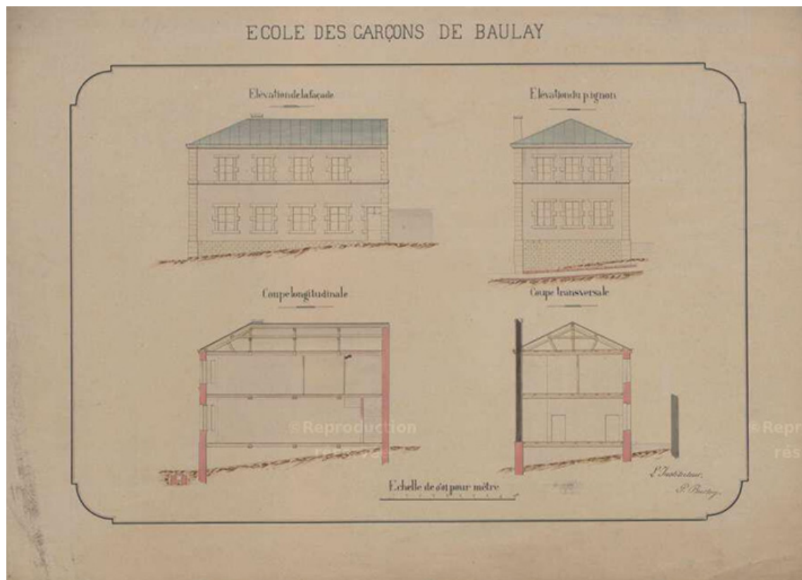
Plans de l'école des garçons 70, Baulay rue de l'Église
