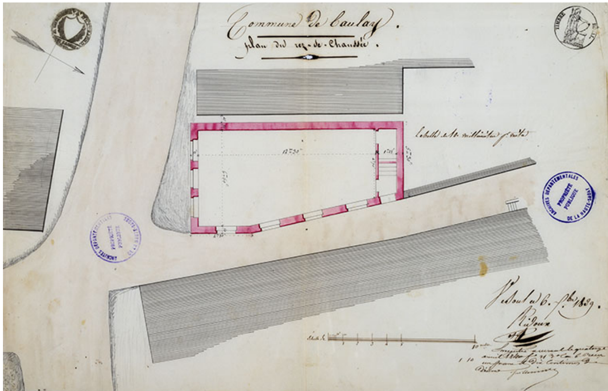
Plan en coupe du rez-de-chaussée de la maison commune, 1839 70, Baulay rue de l'Église
