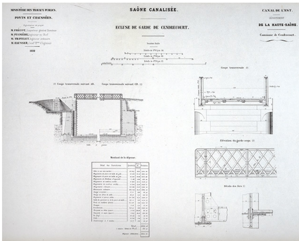
Dessin : Coupe, élévation et détail de l'écluse de garde de Cendrecourt. (1880) 70, Cendrecourt, lieudit : le Closey
