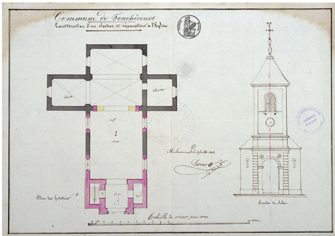
Projet de construction d'un clocher à l'église, plan des fondations (1843). 70, Fouchécourt rue de l'Église
