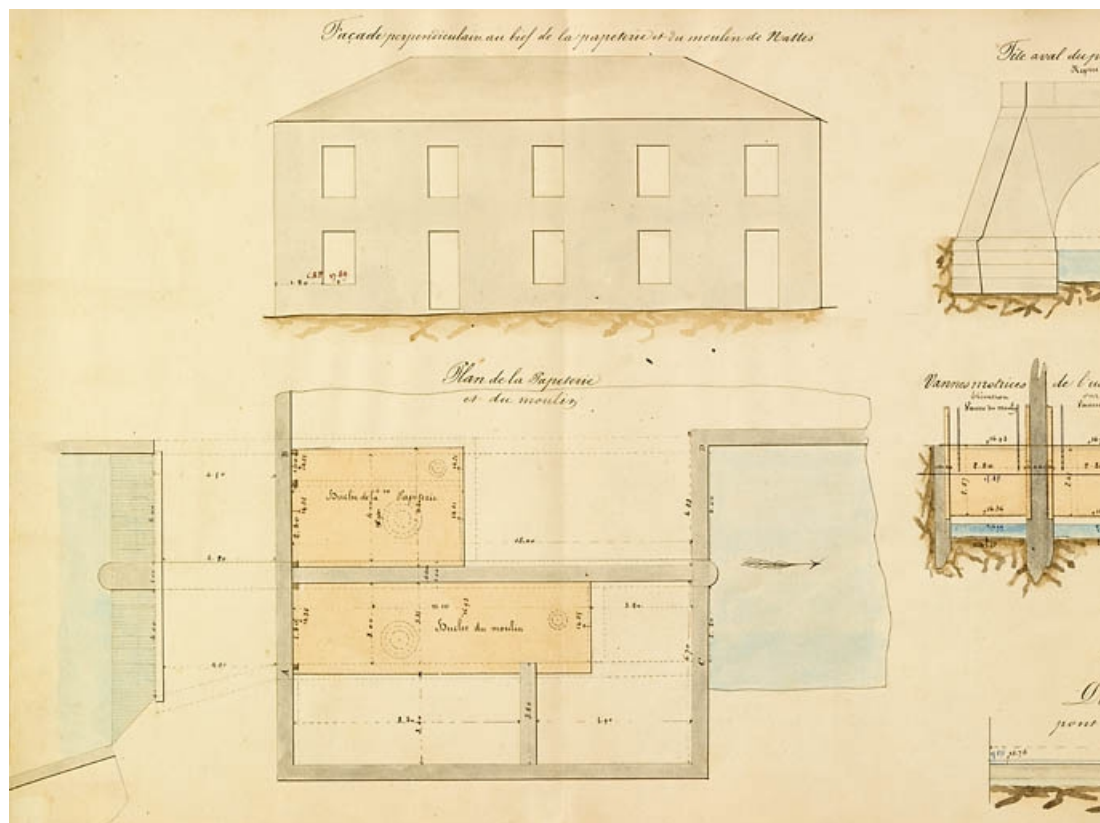
Profils. Plan de la papeterie et du moulin et façade perpendiculaire au bief. 70, Montbozon, 6 rue Bressot
