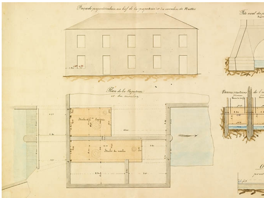
Profil. Plan de la papeterie et du moulin et façade perpendiculaire au bief. 70, Montbozon, 6 rue Bressot
