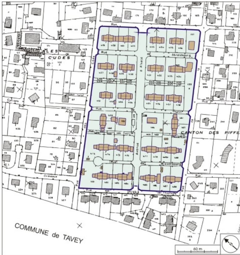
Plan-masse et de situation. Extrait du plan cadastral numérisé, 2005, section AS, 1:1000 réduit à 1:2000. 62, Héricourt rue des Cités Dollfus
