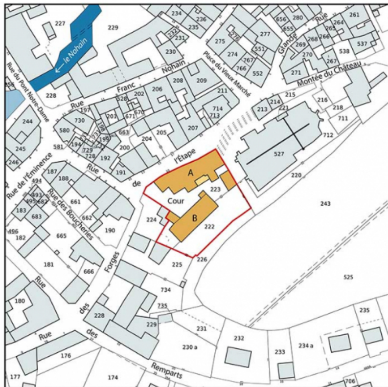
Plan-masse et de situation. Source : Direction générale des Finances Publiques - Cadastre ; mise à jour 2024, section AP, 1/1 000. 58, Donzy, 10 rue de l'Étape
