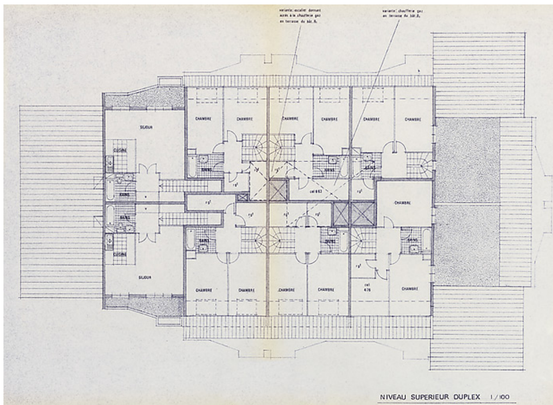
Opération de 132 logements : plan du dernier étage des duplex des immeubles ; F. Martin Lavigne, D. Chenut, O. Senly, septembre 1979. (Archives municipales Cosne-Cours-sur-Loire, 200 W 115 - PC 684)
