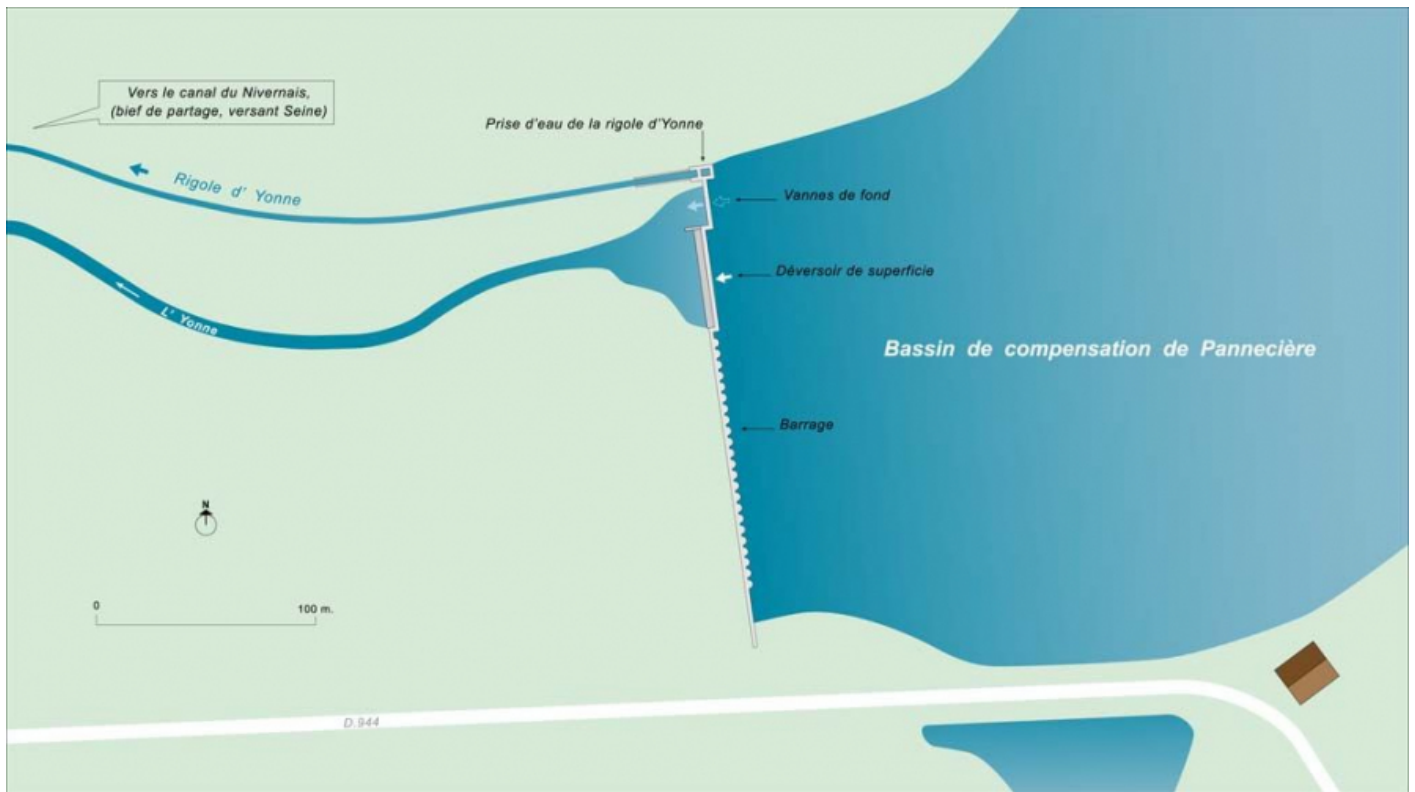
Carte schématique du bassin de compensation et de la prise d'eau de la rigole d'Yonne.
