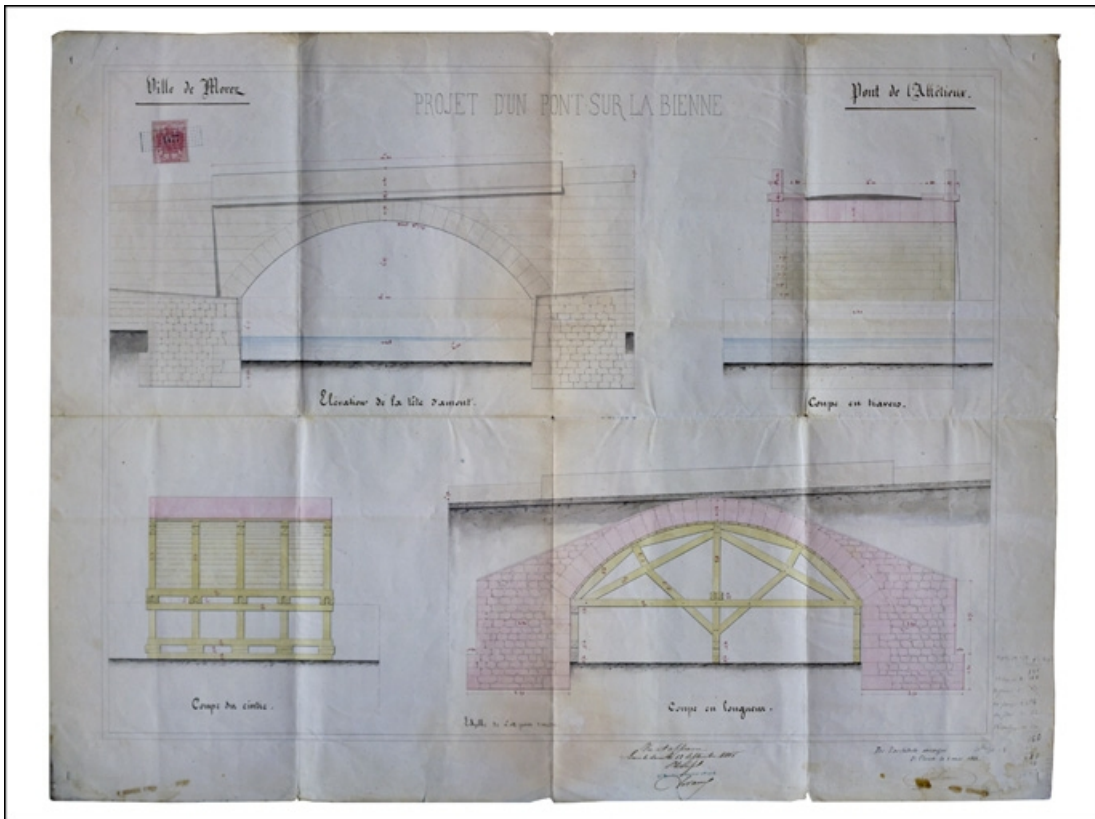
Projet d'un pont sur la Bienne. Pont de l'Affaitieux [élévation amont et coupes], 1866. 39, Morez rue de l' Evalude
