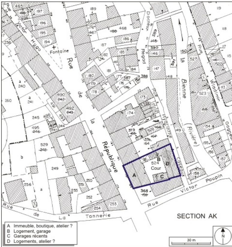
Plan-masse et de situation. Extrait du plan cadastral, 1980, section AI, échelle 1:1000. 39, Morez, 187, 189 rue de la République
