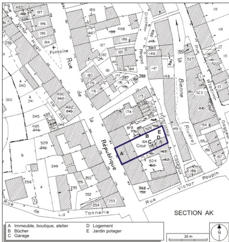
Plan-masse et de situation. Extrait du plan cadastral, 1980, section AI, échelle 1:1000. 39, Morez, 185 rue de la République
