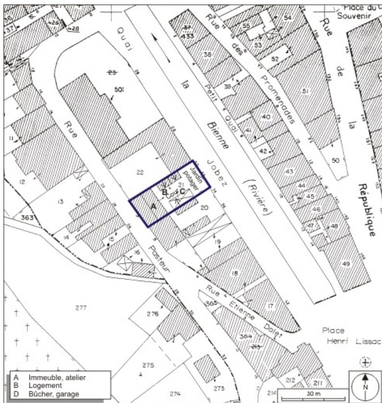
Plan-masse et de situation. Extrait du plan cadastral, 1980, section AI, échelle 1:1000. 39, Morez, 3 rue Pasteur
