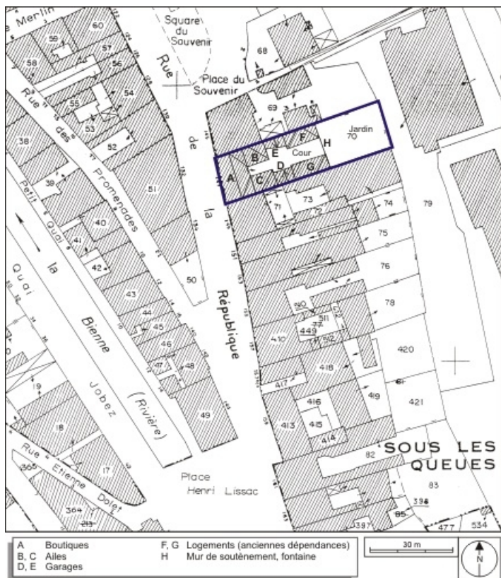
Plan-masse et de situation. Extrait du plan cadastral, 1980, section A1, échelle 1:1000. 39, Morez, 147 rue de la République
