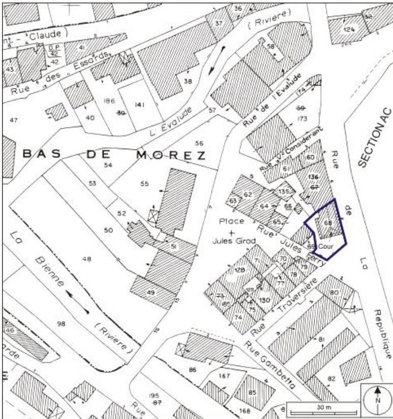
Plan-masse et de situation. Extrait du plan cadastral, 1980, section AB, échelle 1:1000. 39, Morez, 8 rue de la République
