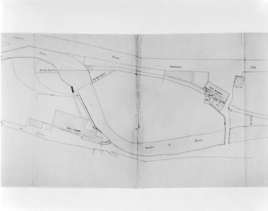
Suppression de l'usine Thievenin Zéphirin de Morez [...] Plan des lieux [détail].
