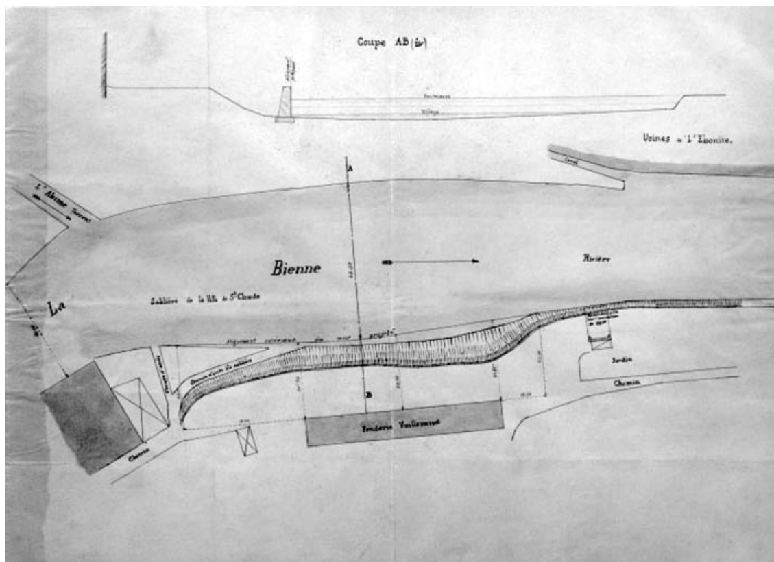
Construction d'un mur [...] Plan et coupe transversale.
