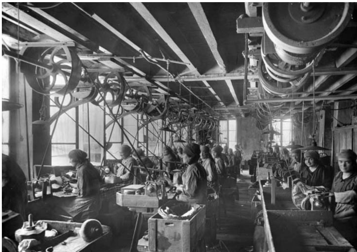
Intérieur de l'atelier de polissage.
