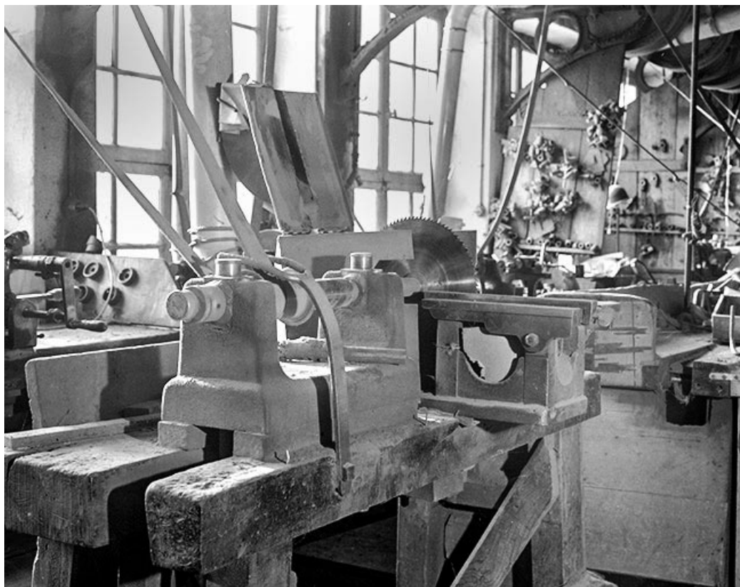
Atelier d'ébauchage : scie circulaire.
