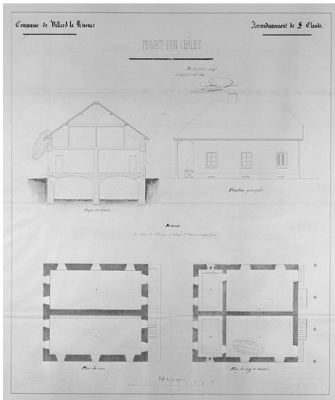
Projet d'un chalet : plan du rez-de-chaussée et des caves, façades, coupes. 39, Villard-sur-Bienne Vallée
