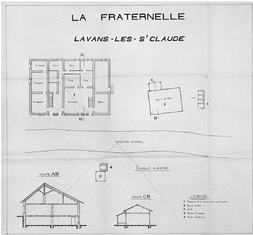
La Fraternelle. Lavans-les-Saint-Claude [plan du rez-de-chaussée et coupe]. 39, Lavans-lès-Saint-Claude, 9 rue de la Cueille
