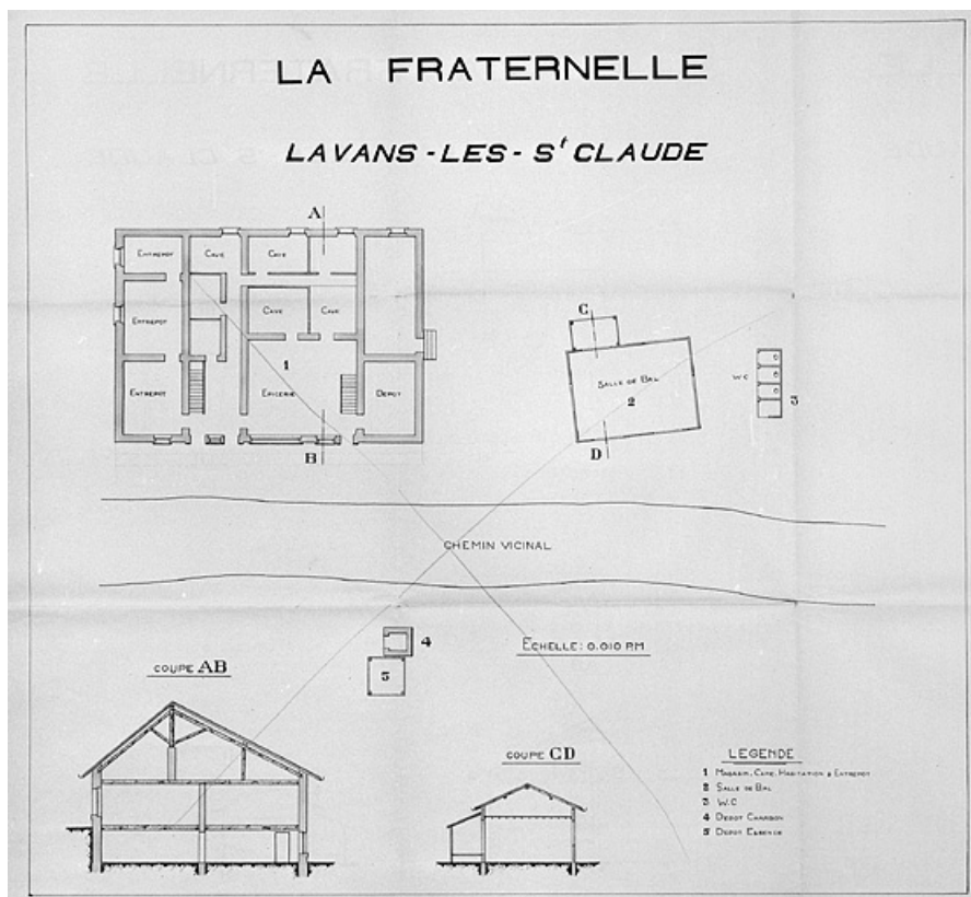
La Fraternelle. Lavans-les-Saint-Claude [plan du rez-de-chaussée et coupe]. 39, Lavans-lès-Saint-Claude, 9 rue de la Cueille
