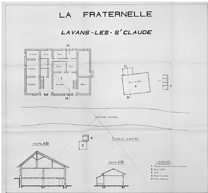
La Fraternelle. Lavans-les-Saint-Claude [plan du rez-de-chaussée et coupe]. 39, Lavans-lès-Saint-Claude, 9 rue de la Cueilie
