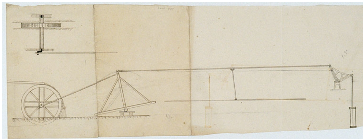
Pompe verticale et son système moteur (roue en dessus, balancier et bras de transmission).
