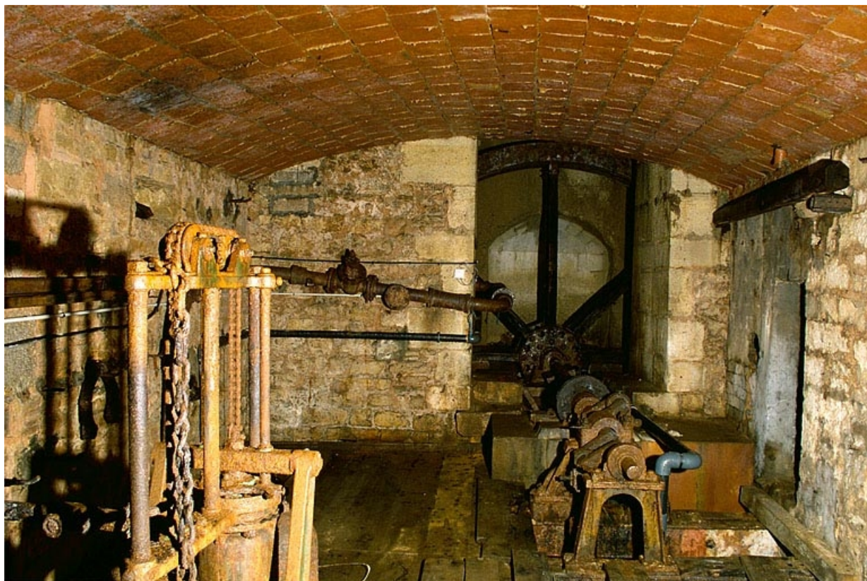
Plancher supérieur du puits à Muire. La roue hydraulique, visible au fond, actionnait une pompe située au fond du puits. 39, Salins-les-Bains place des Salines
