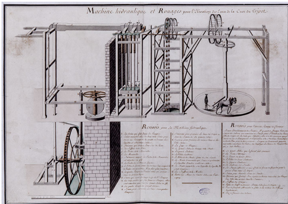
Machine hydraulique et rouages pour l'élévation des eaux de la cuve du Tripot.
