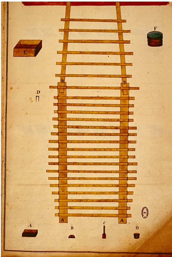
Charpente qui Soutien la Poële et le poëlon.
