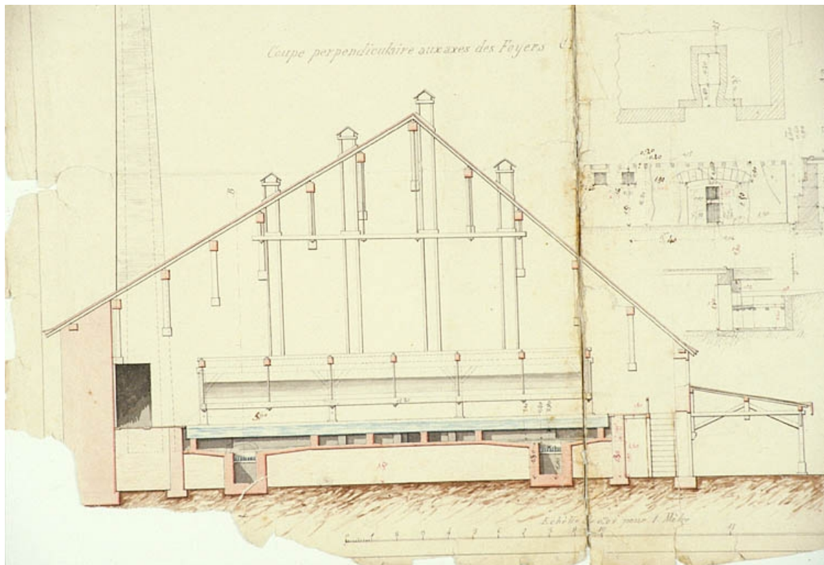
Saline de Salins. Etablissement de deux nouvelles Poêles. Poêle n° 5 [détail : coupe perpendiculaire aux axes des foyers]. 39, Salins-les-Bains place des Salines
