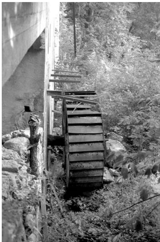
Roue hydraulique verticale amont. 39, Villards-d'Héria
