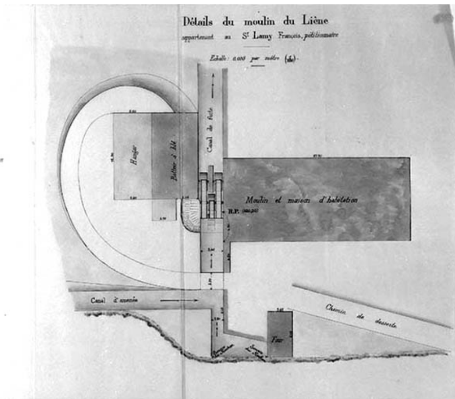
Règlement d'eau [...] Plan et dessins de détails [plan-masse du moulin].
