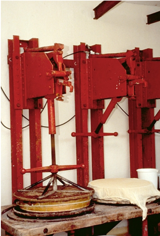
Presses à vis.
