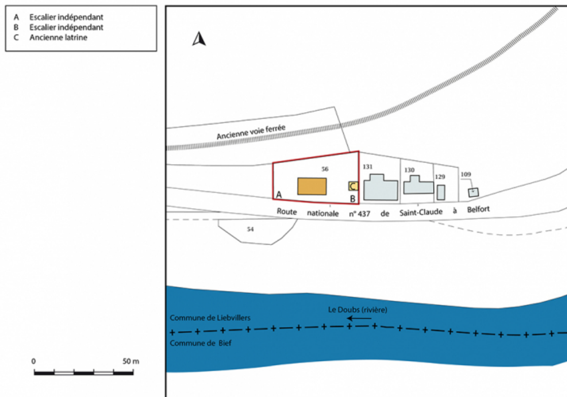
Plan-masse et de situation. Extrait du plan cadastral, 2019, section B. 25, Liebvillers, lieudit : le Gouffre du Lods
