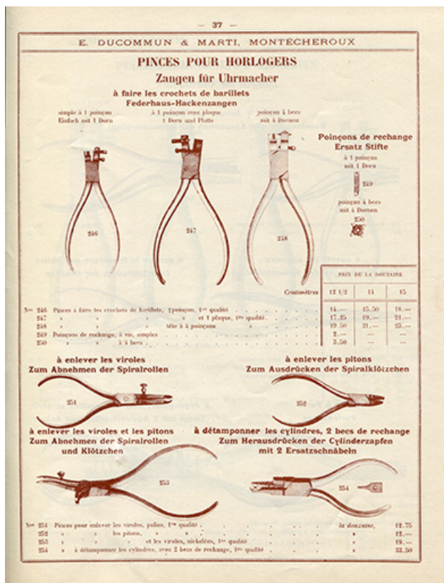
Tarif-album [...] E. Ducommun & Marti successeurs [catalogue de production, p. 37 : pinces pour horloger], [années 1920-1930]. 25, Montécheroux, 1-3 rue de la Planchette
